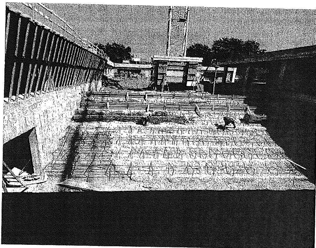
Fig 3. Laje da Bancada Exterior
